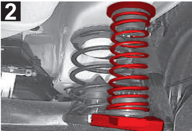
2 Tra il ponte della ruota e la carrozzeria - Between the rear axle and chassis - Zwischen Achse und Karosserie - Entre le pont arrière et la carrosserie - Sobre el puente de la carroceria Tussen de achteras en chassis
