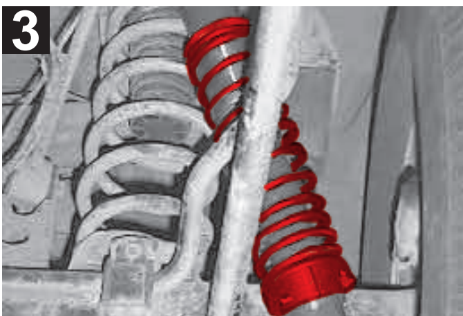
3 Sull'ammortizzatore nel tipo UNIVERSAL - On the shock absorber using a UNIVERSAL spring - Auf dem Stossdämpfer (UNIVERSAL) Sur l'amortisseur, avec ressort type UNIVERSAL - En el amortiguador Om de schokbreker
