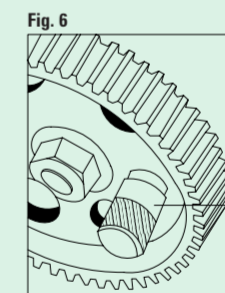
FIGURA 6 Insertar la herramienta para inmovilización de polea de bomba de inyección H.
