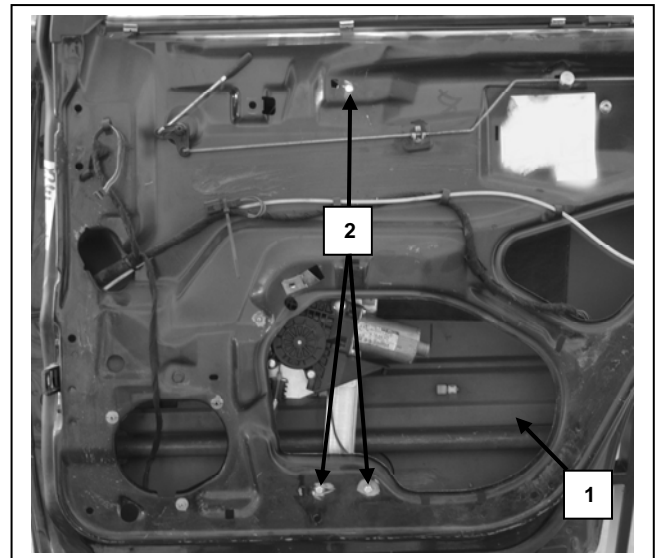
Puerta lado derecho, Right rear door
